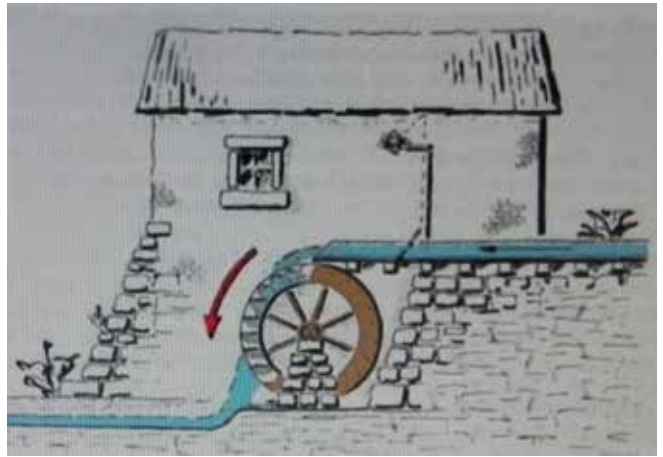
Unterschlächtinge Mühle
